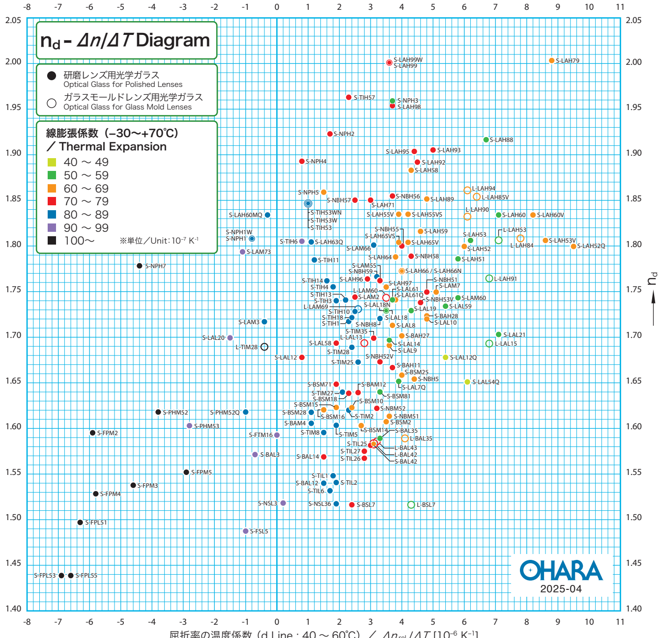
屈折率の温度係数 (d Line; 40 ~ 60°C) / \Delta n_{rel}/\Delta T [10^{-6} \text{ K}^{-1}]
